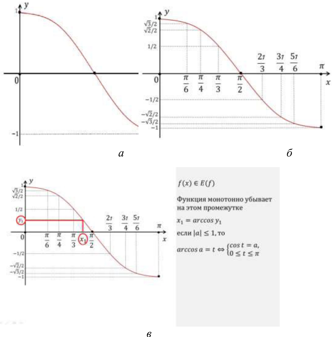
Рис. 2 – Введение понятия арккосинуса
